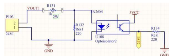
Figura 5. Circuito de etapa de potencia fuentes 24V
